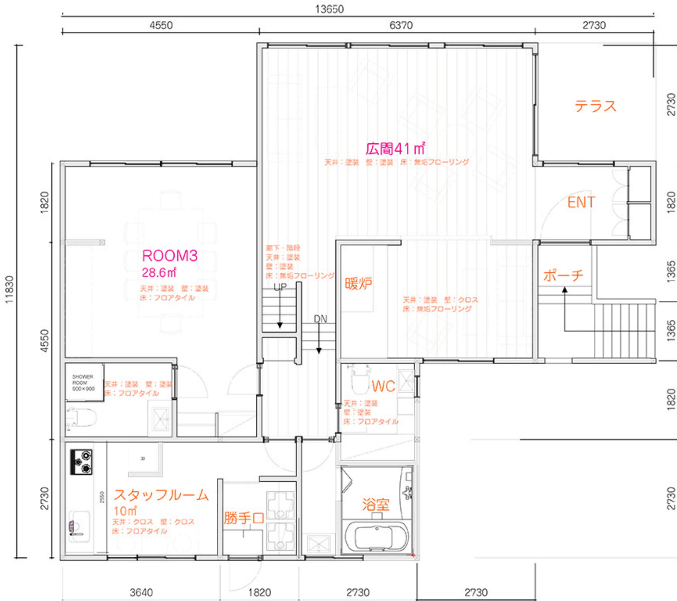
© 1F 平面図 S=50:1
