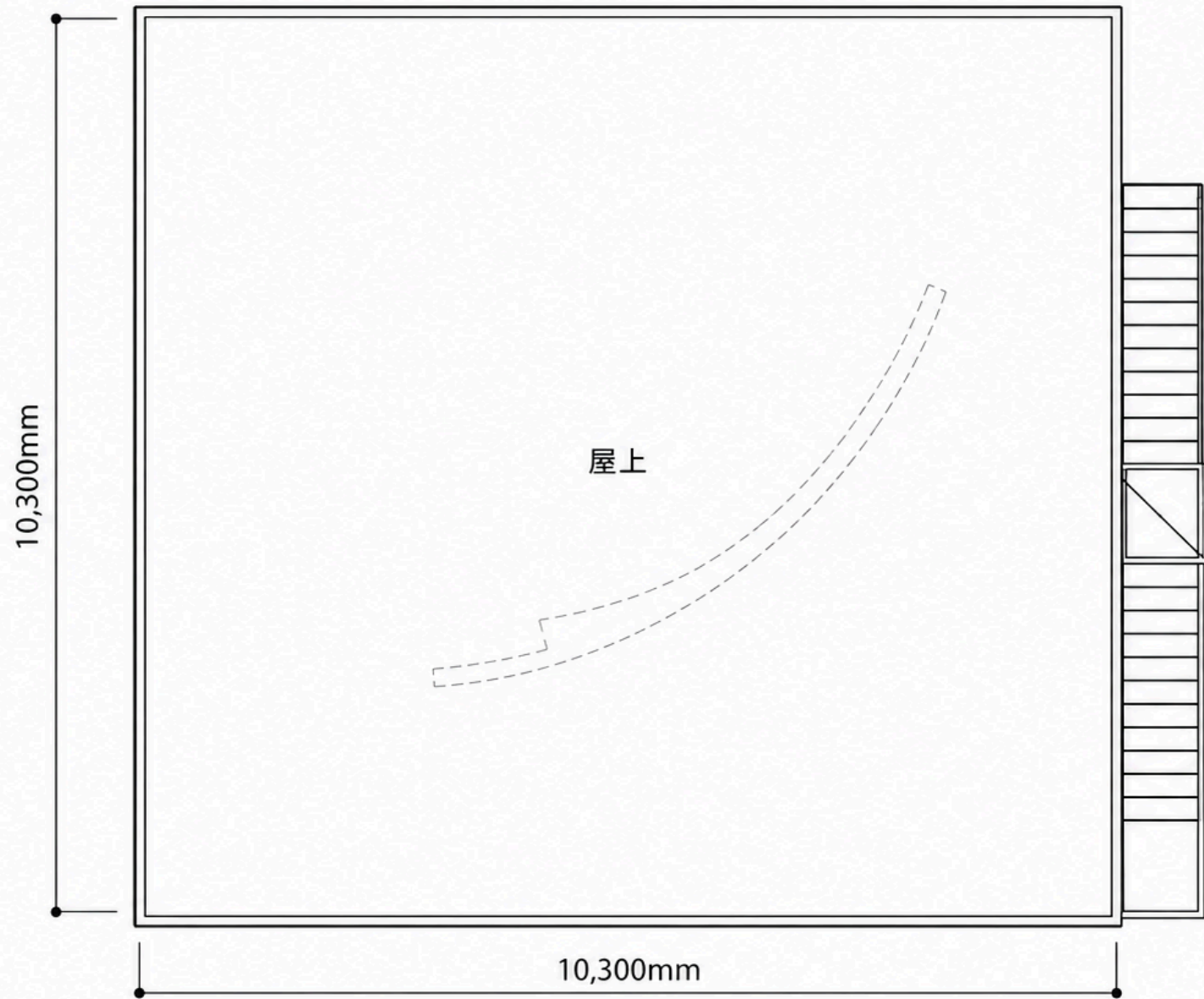
屋上平面図
