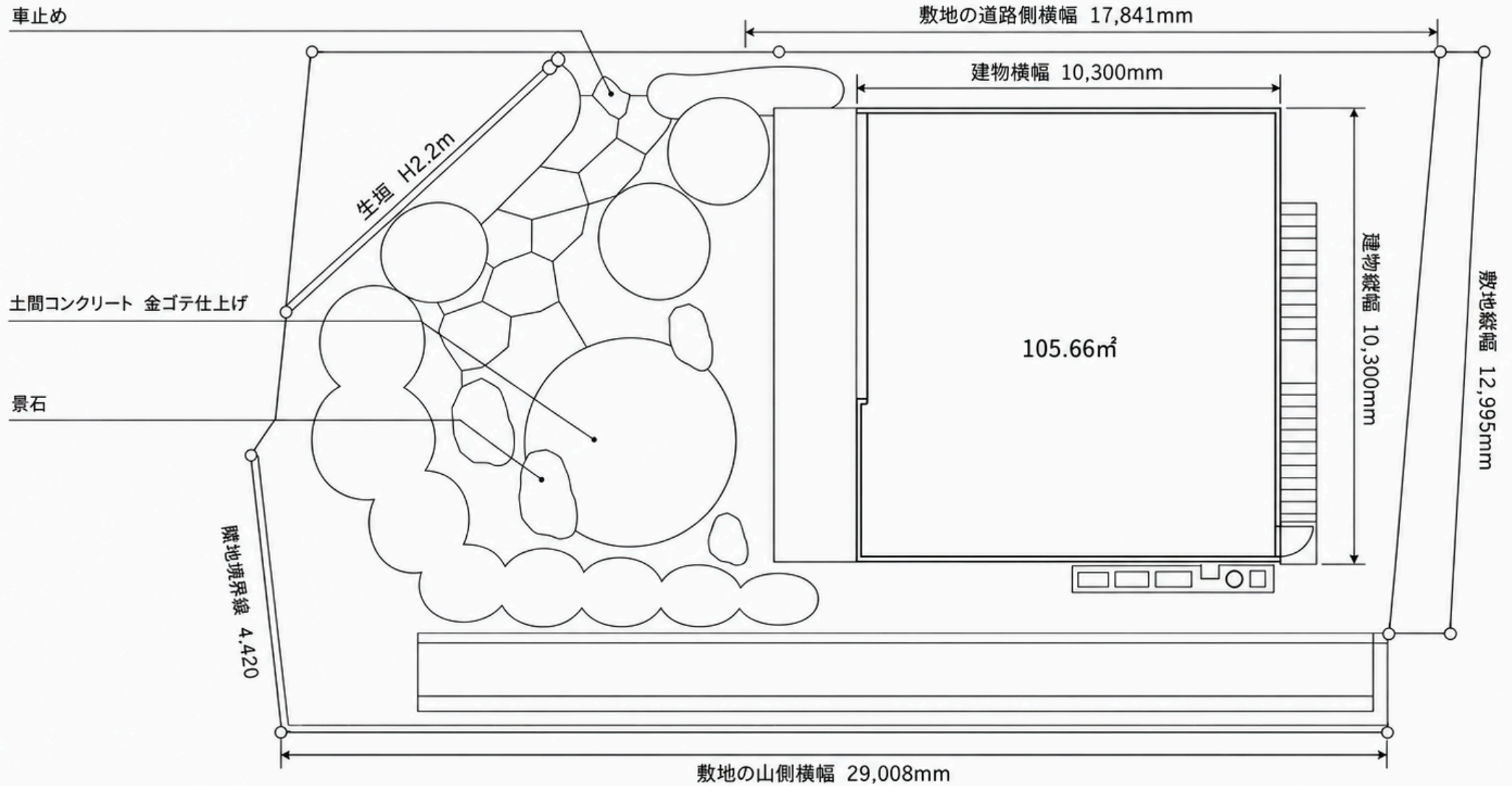
全体平面図
