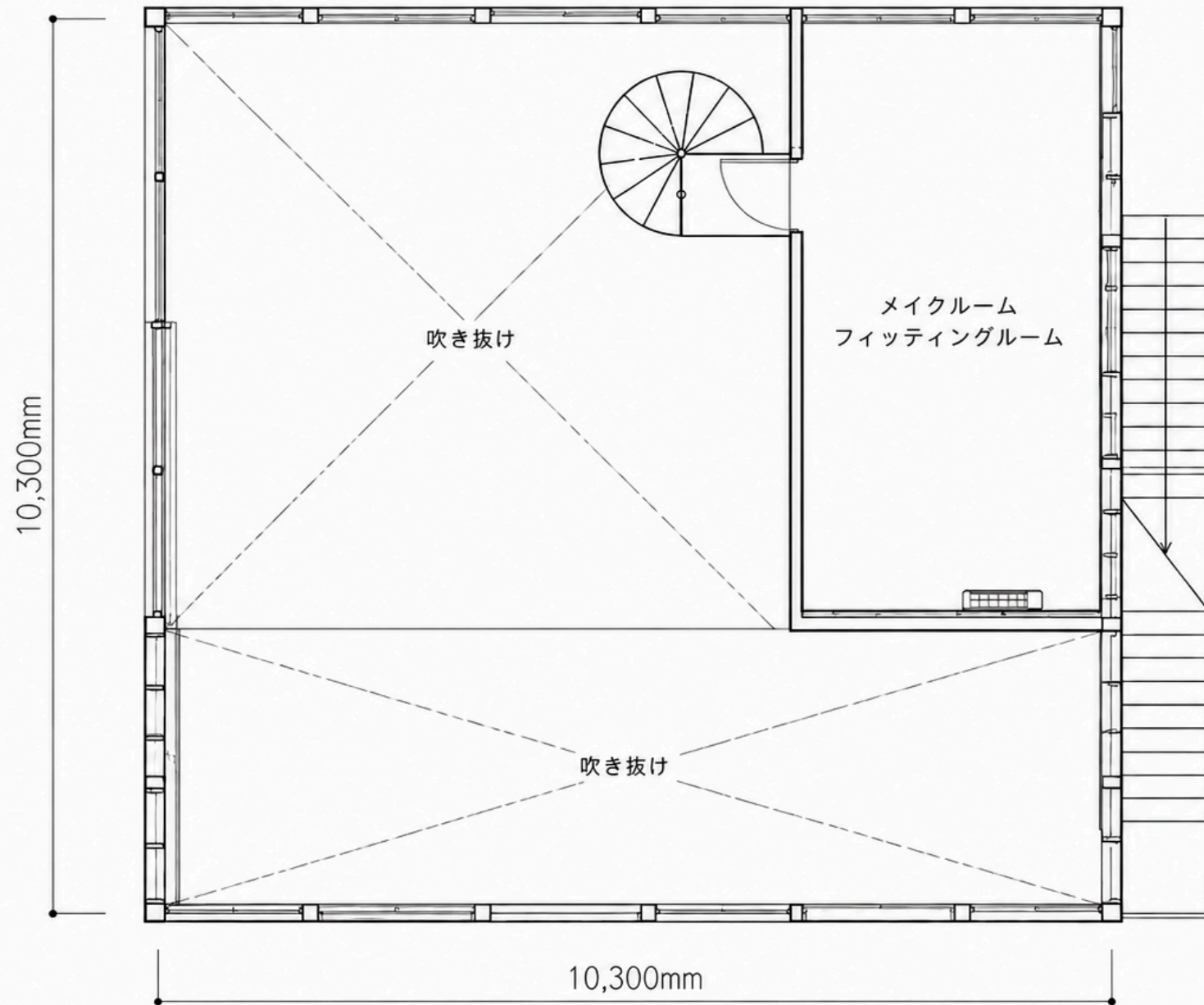
2階平面図
