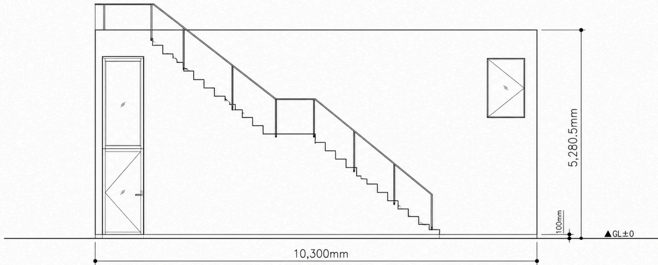
北立面图
